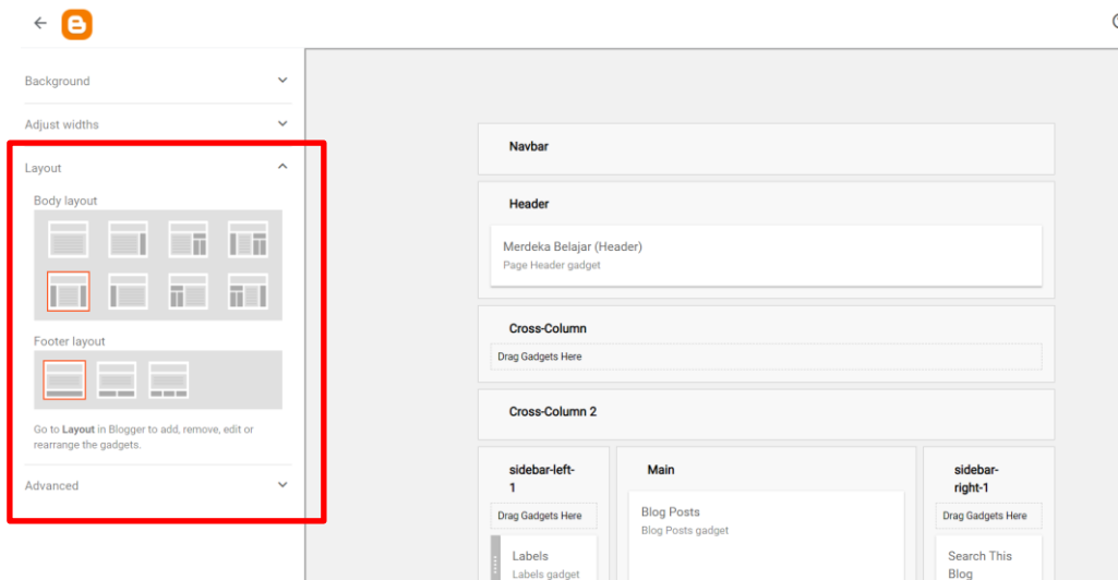
Gambar 5.52. Layout Editing pada Theme Simple
