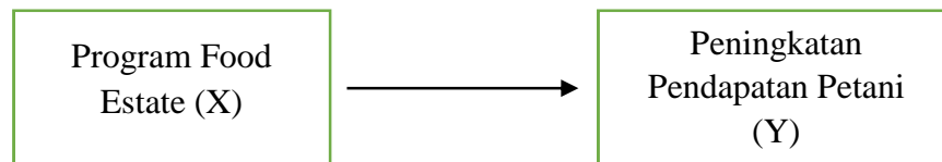
Gambar 2.1 Kerangka Berpikir
