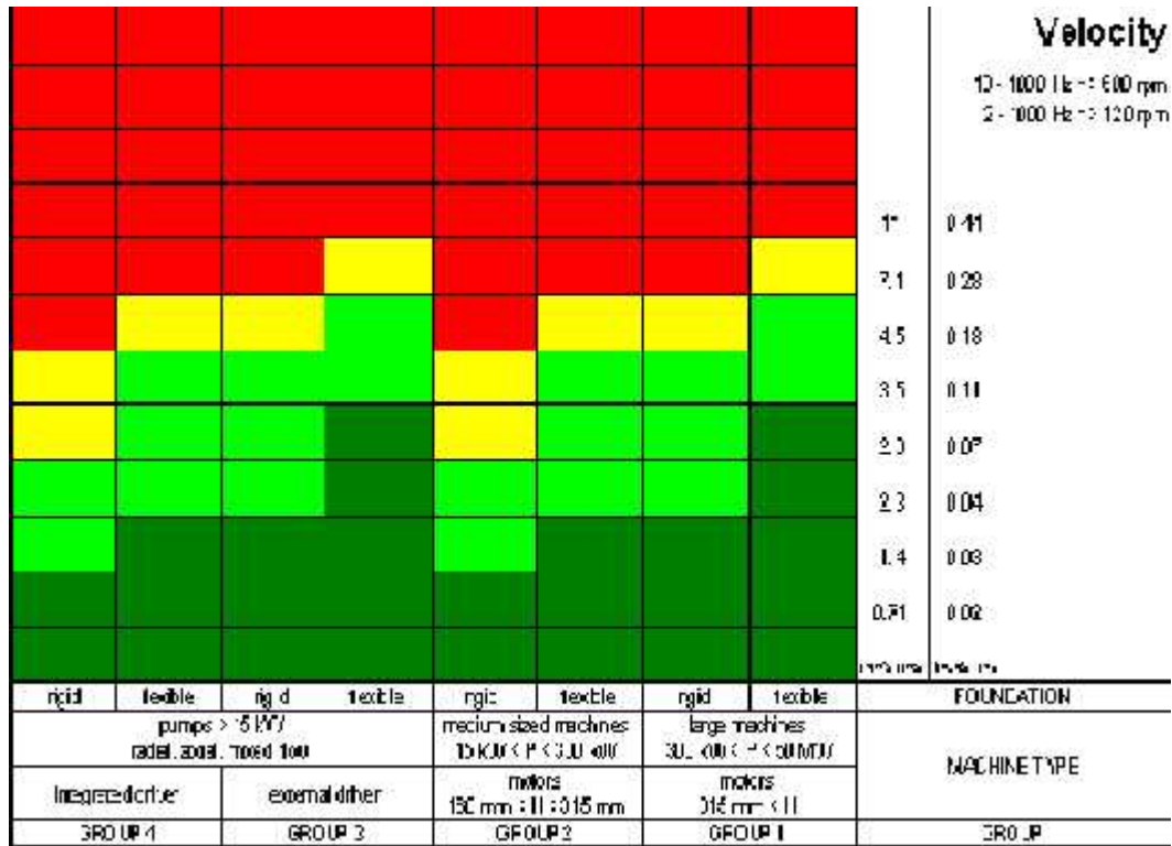
Gambar 1.1 Standart ISO 10816-3 untuk getaran. (Dynaseq. 2006]
